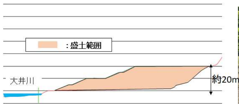
A-A'断面図
