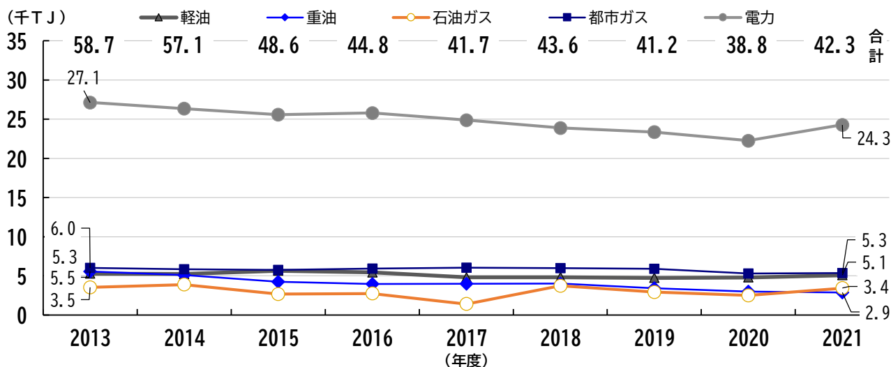
参考図13 業務部門 主なエネルギー消費量の推移
