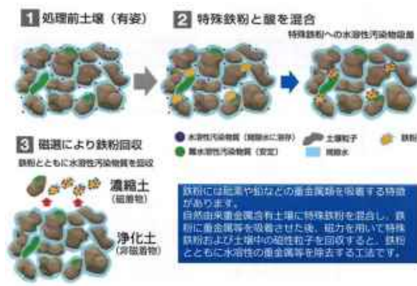
図 26 磁力選別処理の浄化方法
