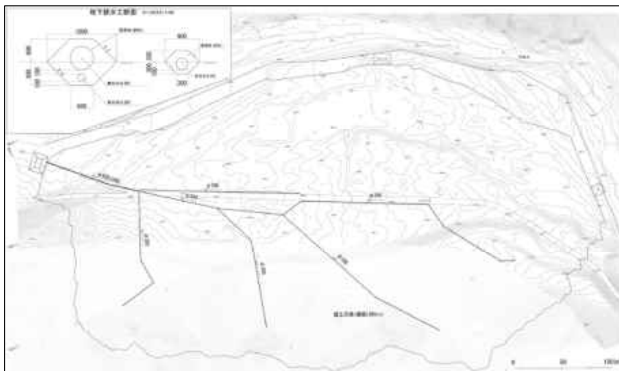
図 18 地下排水敷設図
