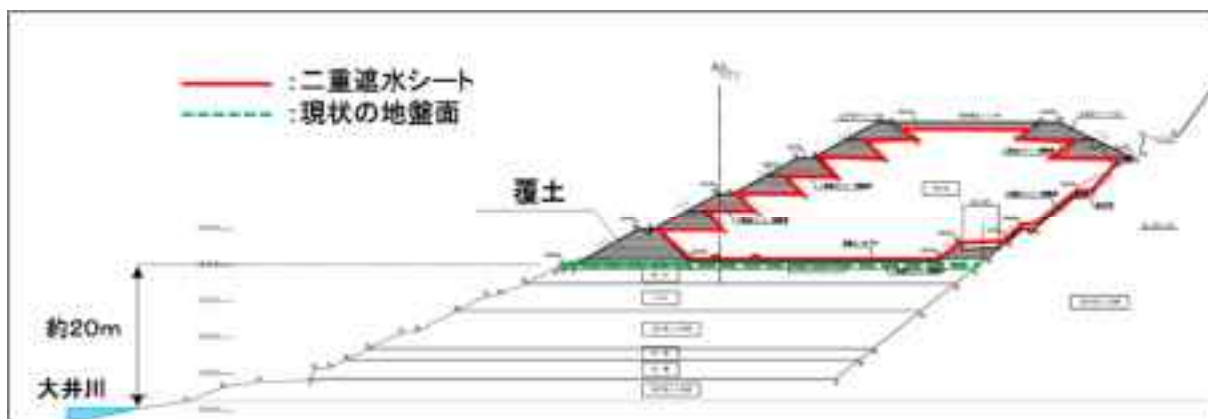
図 2 2 藤島沢付近の発生土置き場（遮水型）横断面図（A－A'断面）
