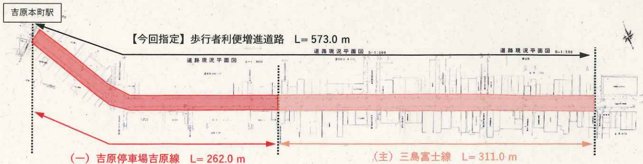
《平面図》
